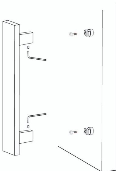
Συναρμολόγηση με βουιδόνι Bolt assembly
