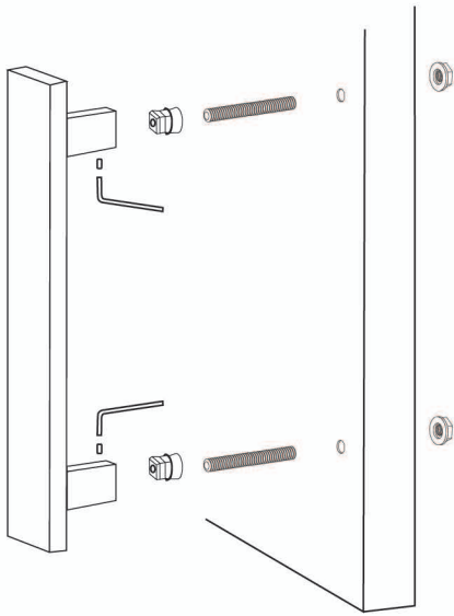
Διαμερής συναρμολόγηση Through Holes assembly
